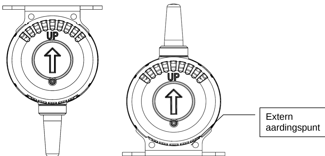
Afbeelding 2-1: Correcte positie van de weerkap en positie van het aardingspunt.
