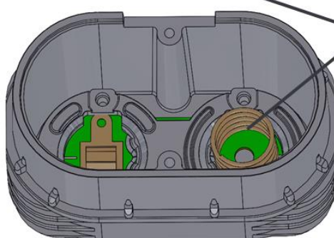
Figur 5-2: Batterihuset sett nedenfra. Korrekt tilkobling av multimeteret.
