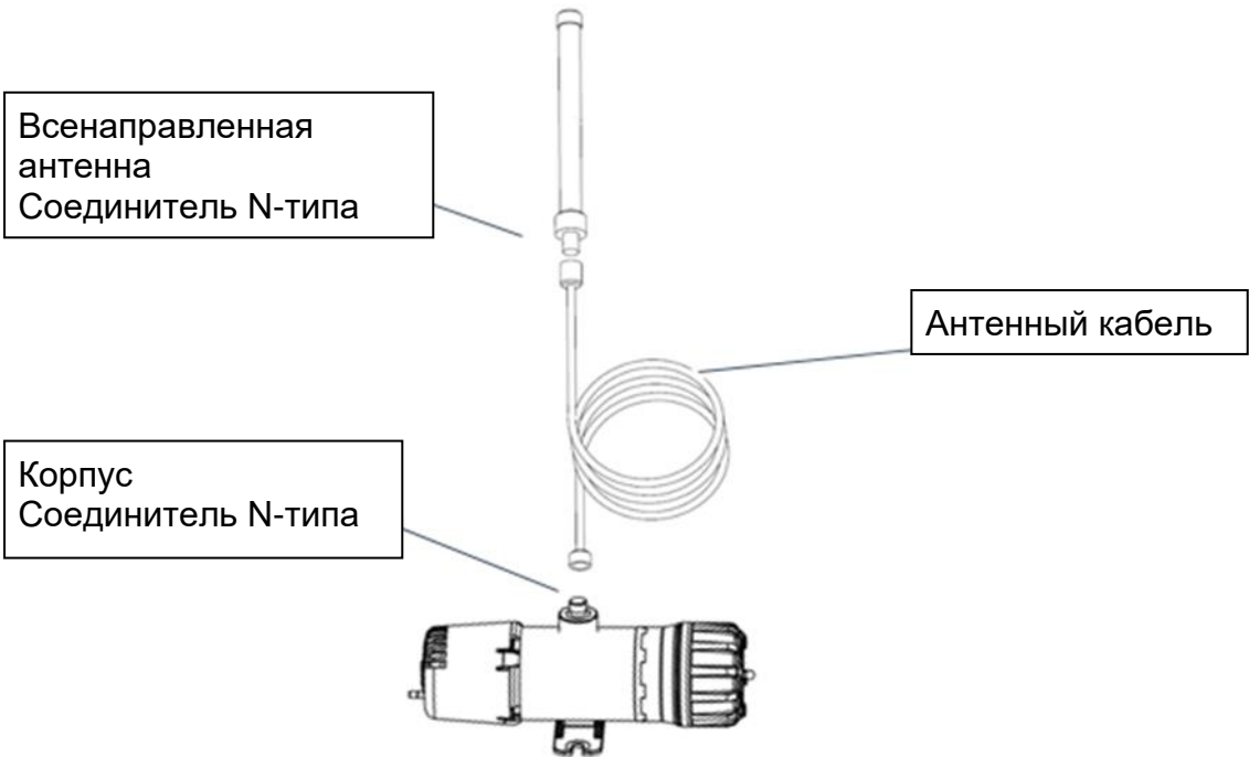
Рис. 2-2: Блок-схема GS01-EA с соединениями антенны
