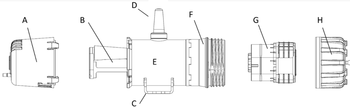
그림 1-1: GS01 겹치기 분해도
