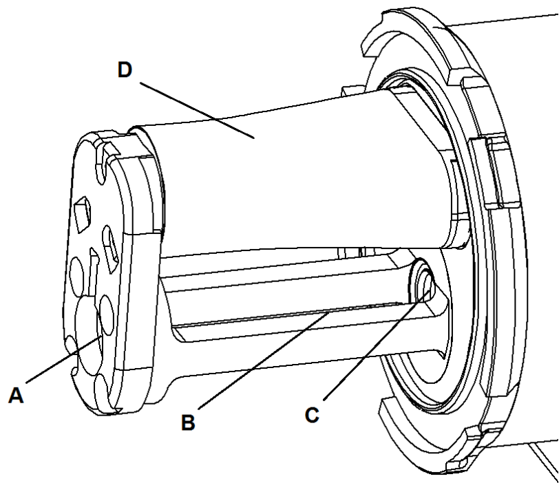
图 1-4: GS01 测量池详细结构
