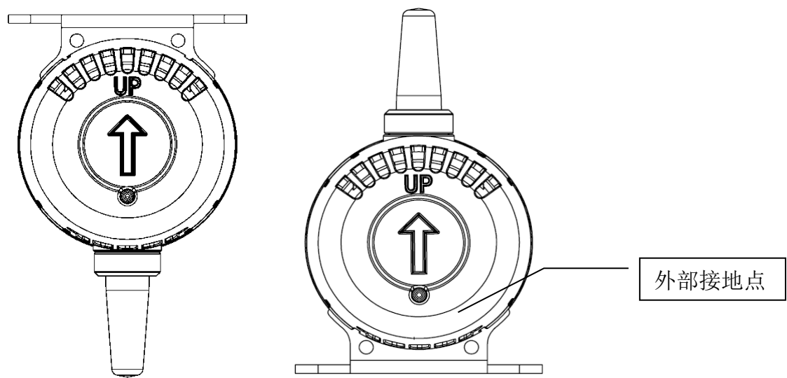
图 2-1：防风罩的正确位置和接地点位置。 无论检测仪的方向如何，箭头都必须始终朝上。
