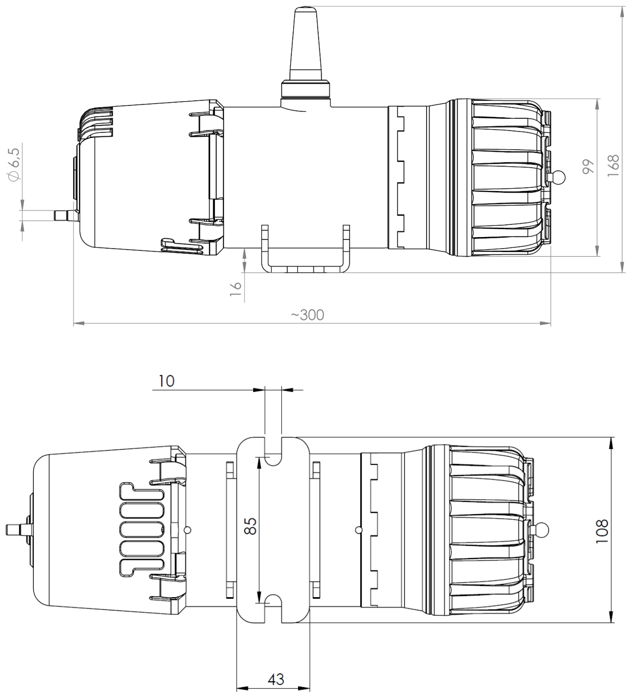
图 1-2: GS01 检测仪尺寸, 单位为[mm]
