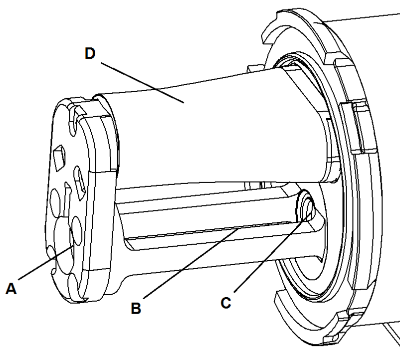
Figura 1-4: Detalles de la célula de medición GS01
