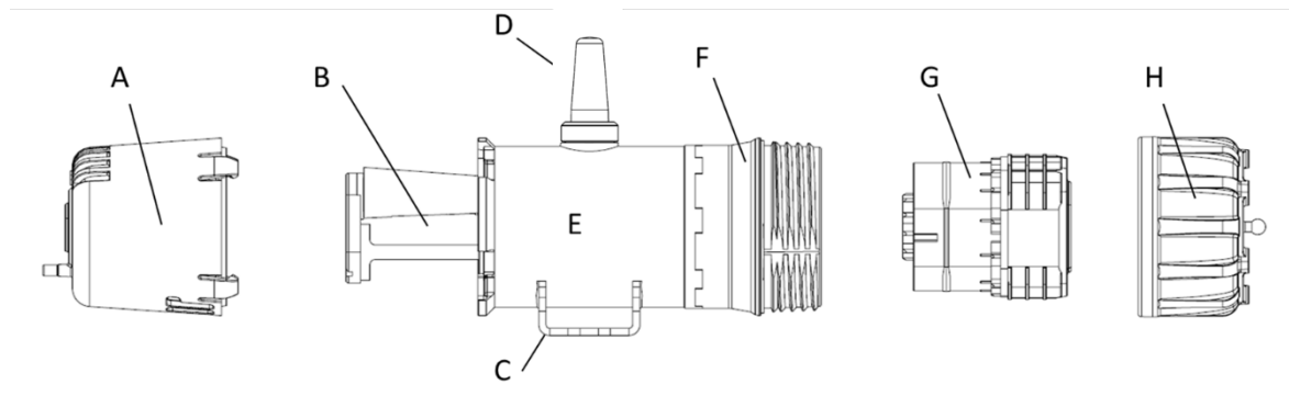
그림 1-1: GS01 감지기 분해도
