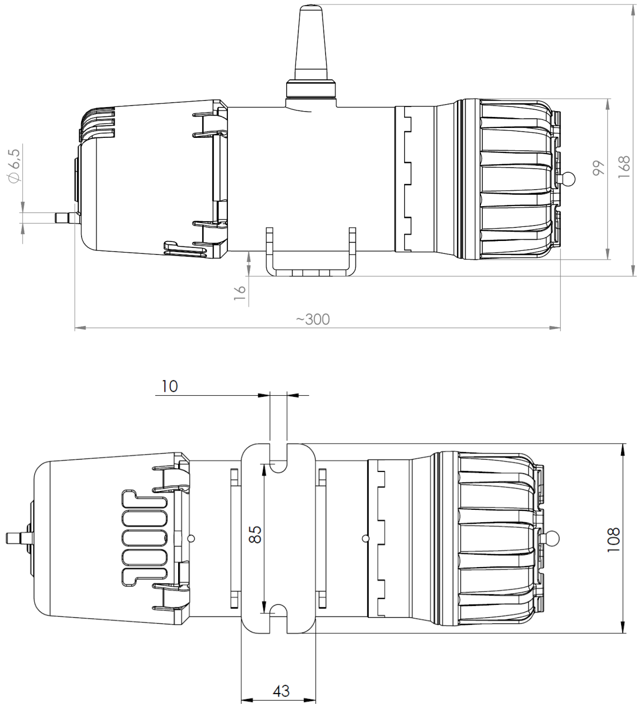
그림 1-2: GS01 검지기 치수도[단위: mm]
