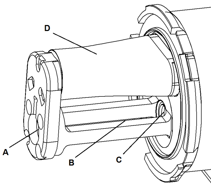
Figura 1-4: Detalhes da célula de medição do GS01
