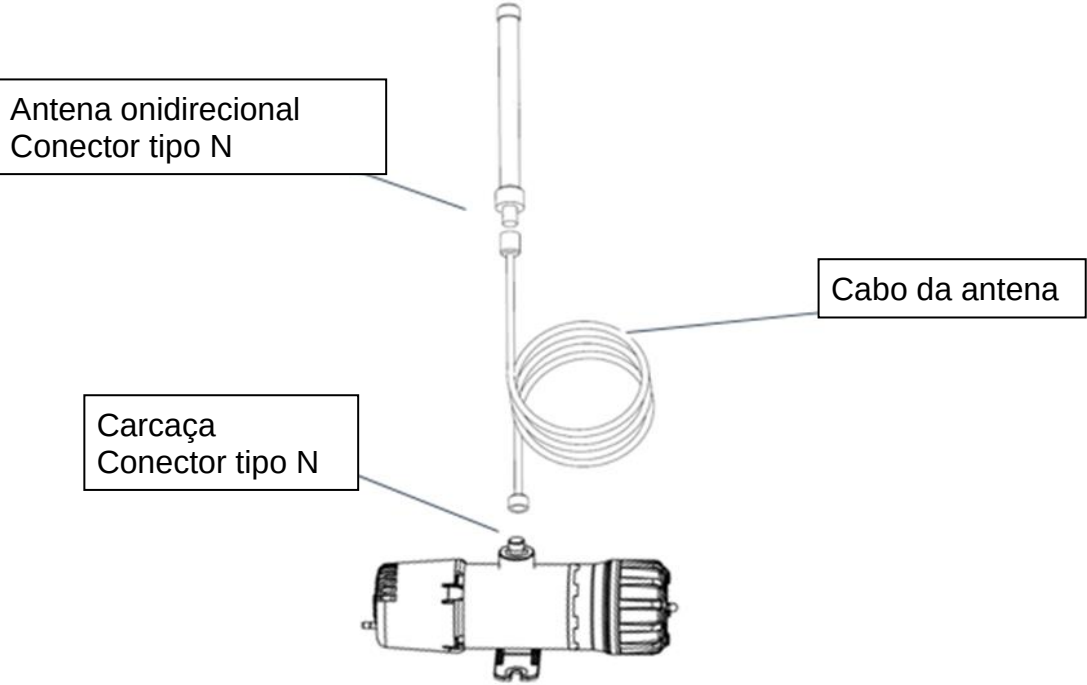
Figura 2-2: Layout do GS01-EA com conexões da antena
