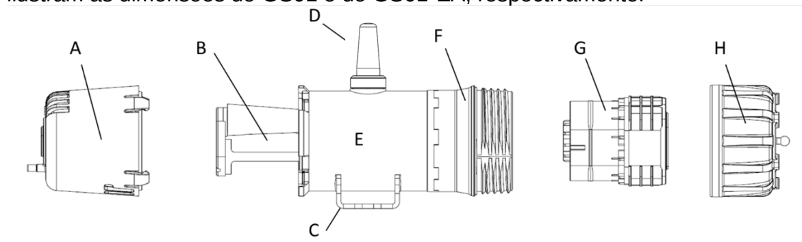
Figura 1-1: Layout do detector GS01
