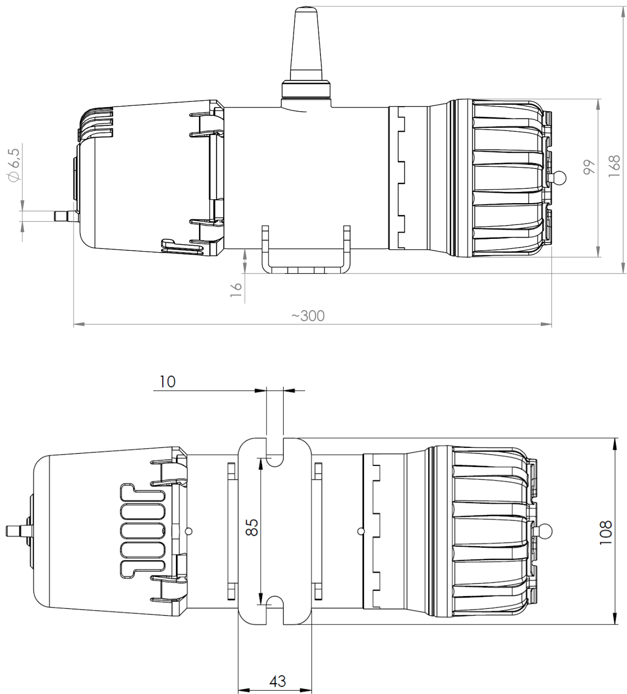
Figura 1-2: Detector GS01 com dimensões em [mm]
