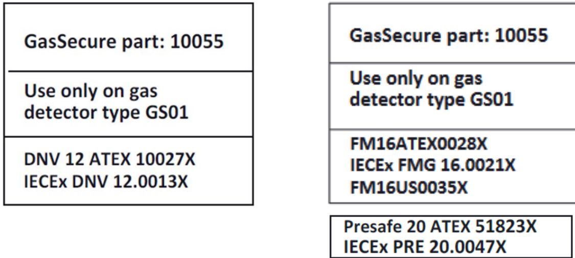
Figura 7-6: Rótulo de identificação do conjunto da bateria (versão aprovada pela FM à direita)
